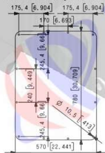
Style A Lid plate Blank Lid
