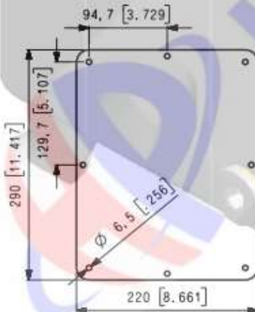
Style A Lid plate Blank Lid
